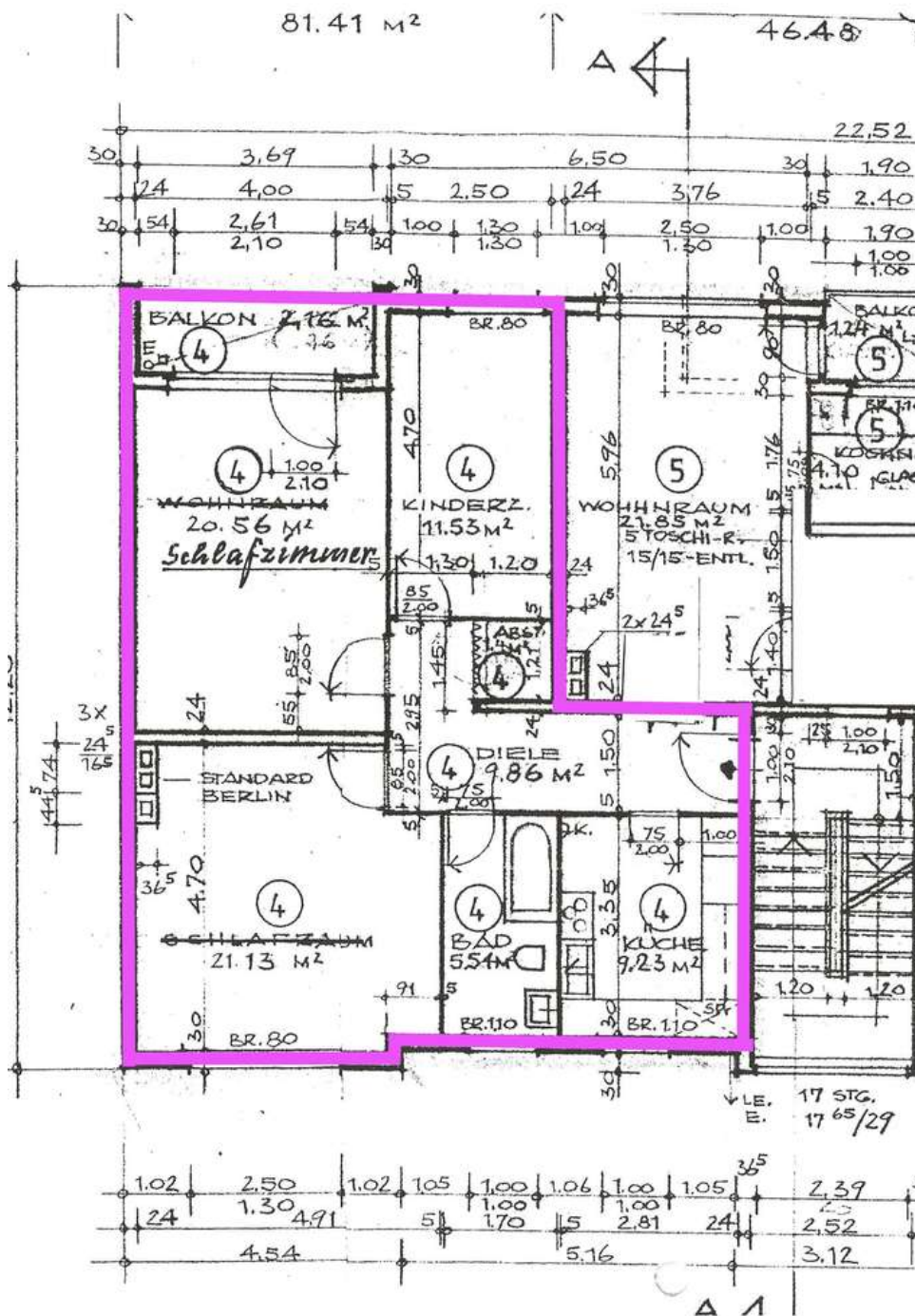
Grundriss WE4
